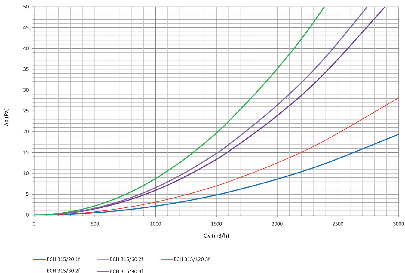
ECH 315
