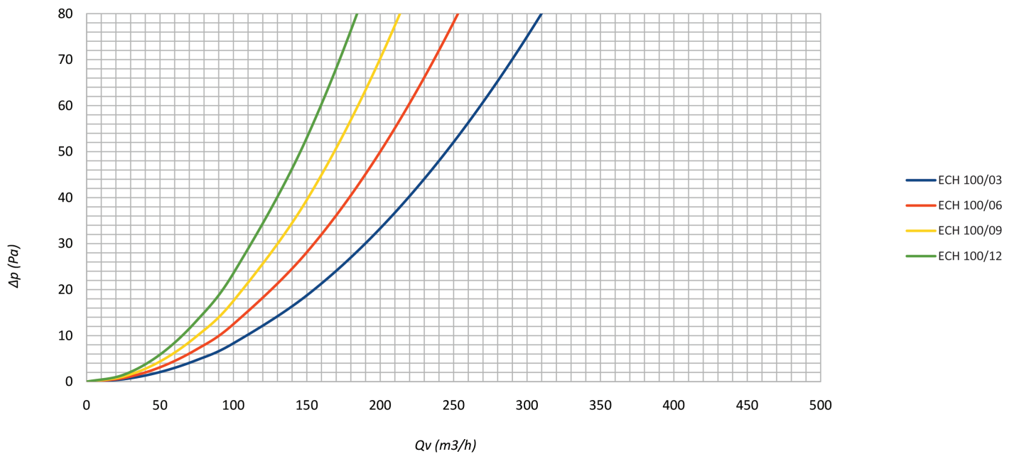
ECH 100
