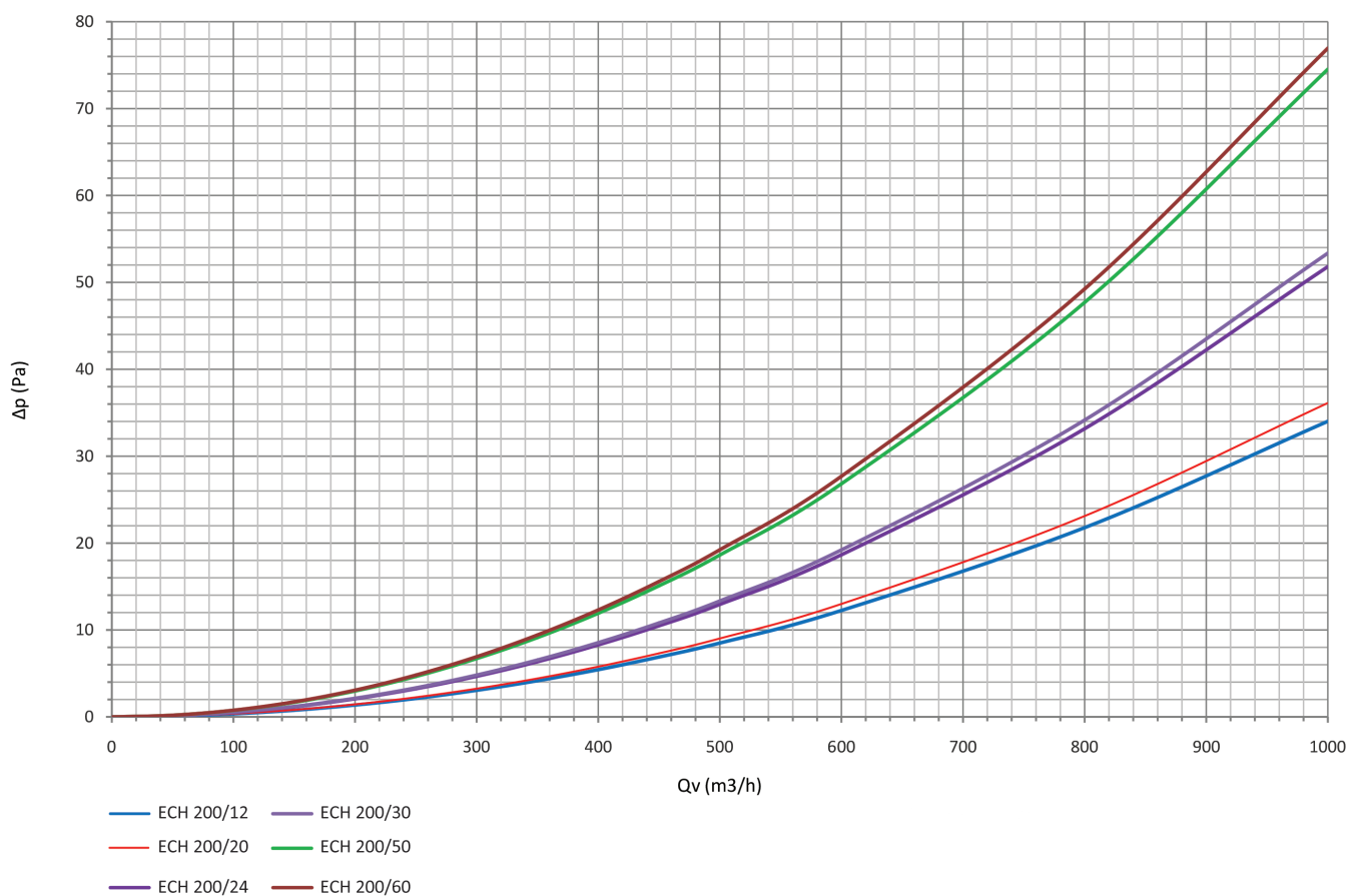
ECH 200
