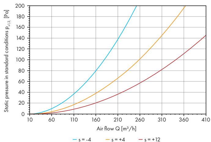
EV-SC 200
