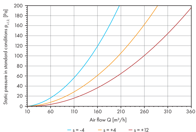
EV-SC 160
